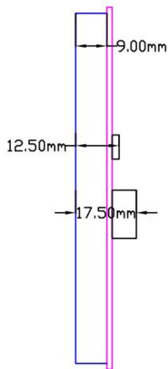
右侧面图
