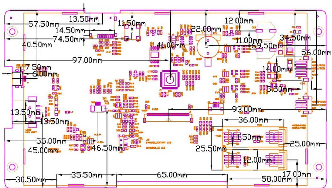
AMZ070 背面图
