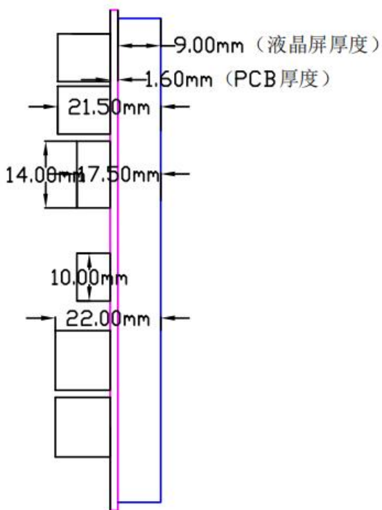
左侧面图
